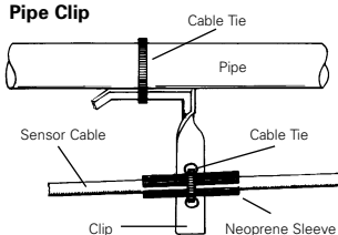
Pipe Clip
